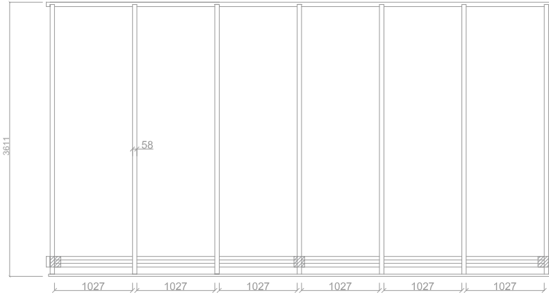
BOVENAANZICHT
