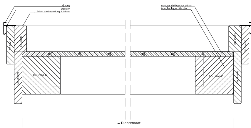
Terrasoverkapping modern vrijstaand doorsnede
